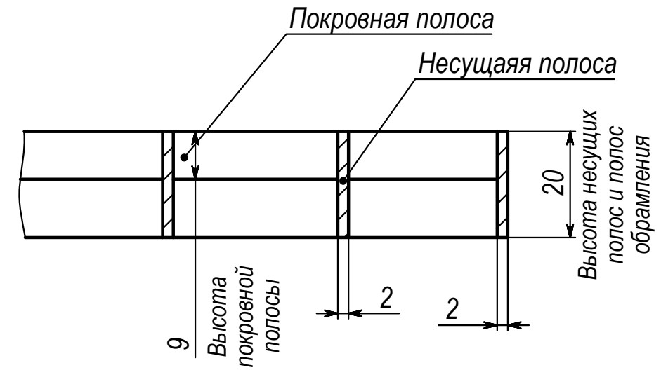
Б-Б (1 : 1)
